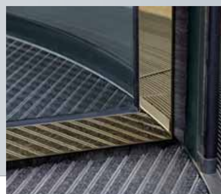
KONTORHAUS GEBR. HEINEMANN KG | HAMBURG | Typ GGG v špeciálnom prevedení | plnoautomatický | krídla dverí opláštěné titanizovanou ušľachtilou oceľou | zrkadlovo leštené | strop plechovej konštrukcie | ø 2860 mm
