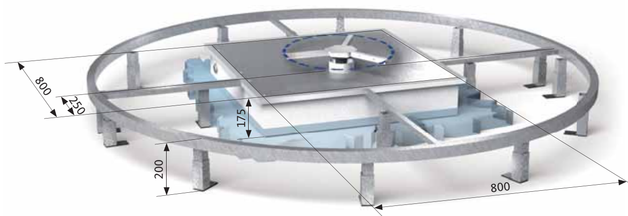
podlahový kruh s podpodlažným pohonom
