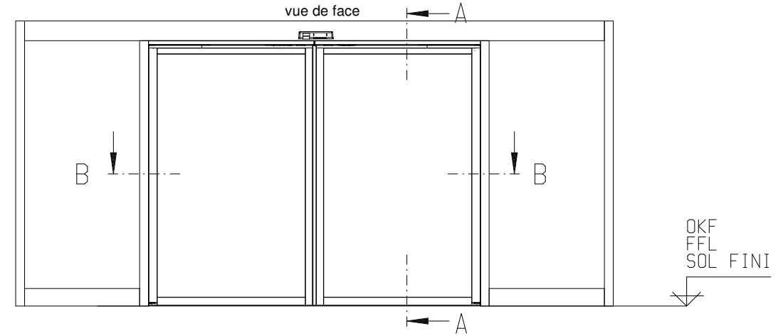
Ansicht Aussen front view vue de face
